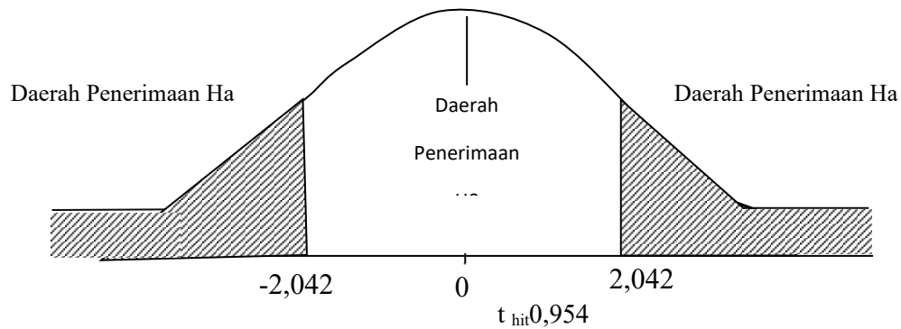
Gambar 2 Kurva penerimaan dan penolakan H_0 ( \alpha )
